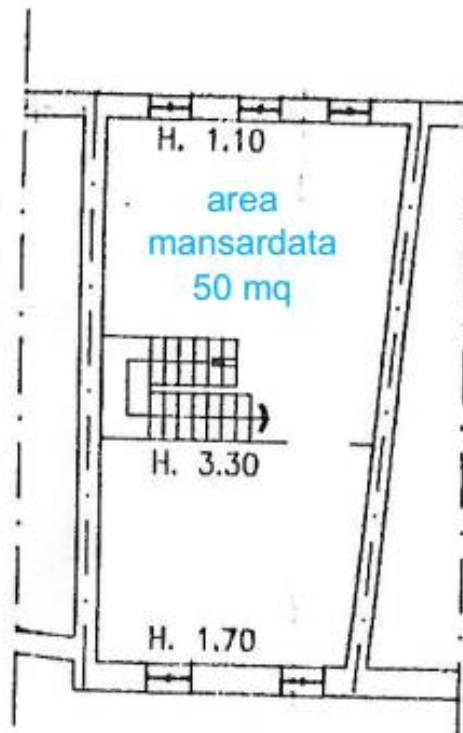
Piano SOTTOTETTO
